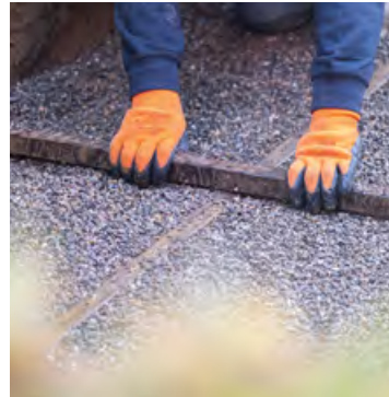
02. Preparación de la base con una solera de grava
