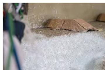
06. Proyectado final con fibra de vidrio y resina exclusiva
